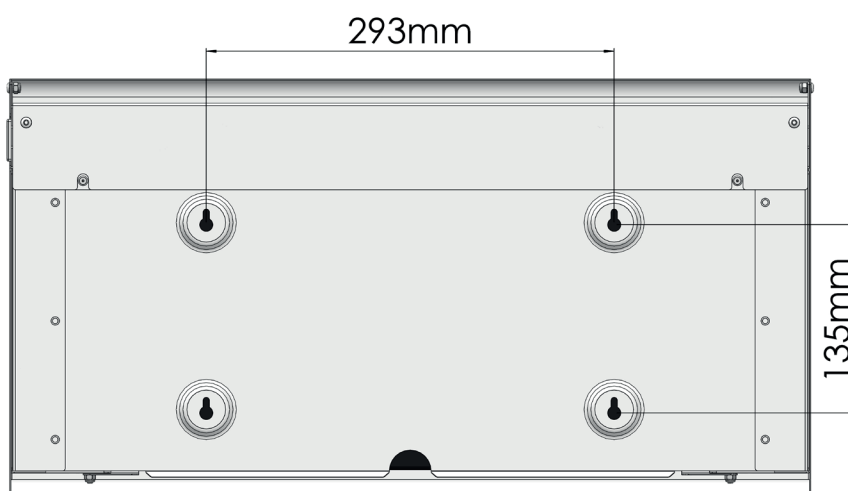
Abbildung 1 - Schlüssellocher zur Wandmontage
