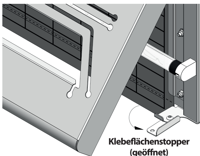
Abbildung 2 - Klebeflächenstopper
